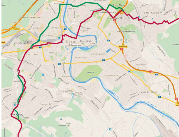
Vorgeschlagener Verlauf der Velohauptachse Köniz-Bern-Ostermundigen: 1. Phase (dunkelrot): Entlang bestehender Neben- und Hauptstrassen. 2. Phase (grün): Mögliche Ausbaumassnahmen.
